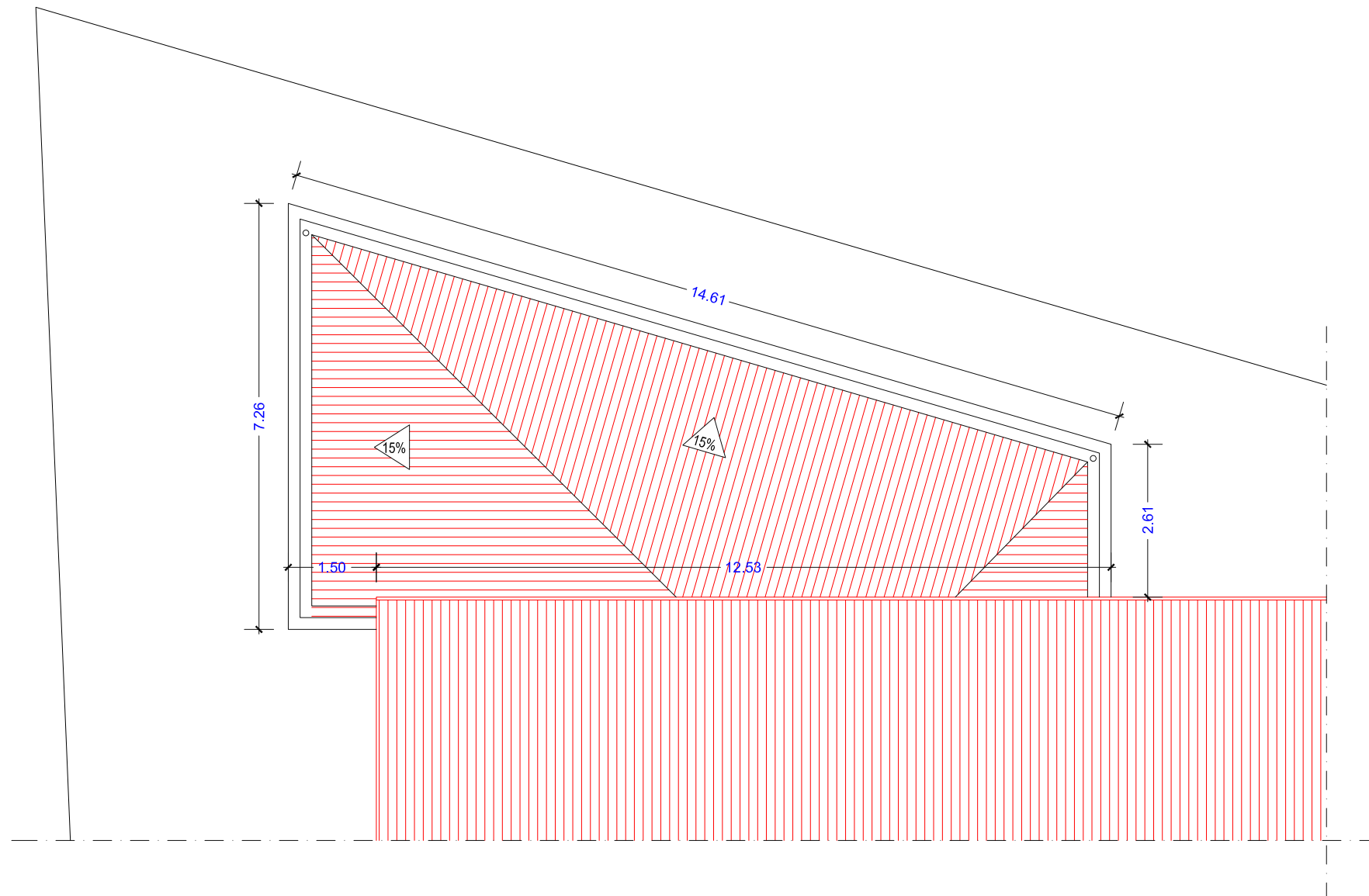
PLANTA DE CUBIERTAS
